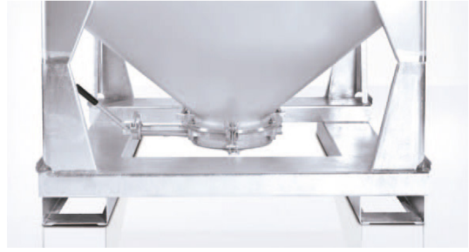
Auslauf: direkt am Flansch angeschraubte Absperklappe mit Handhebel, 60° gekanteter Trichter, verschraubtes Untergestell mit durchgehenden Gabeltunneln.
